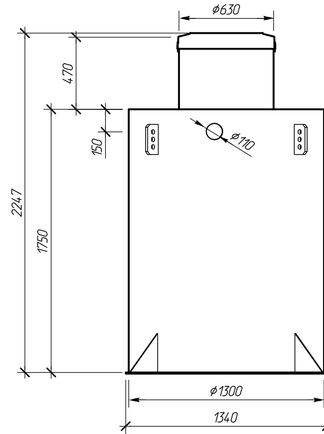
Вид сбоку
