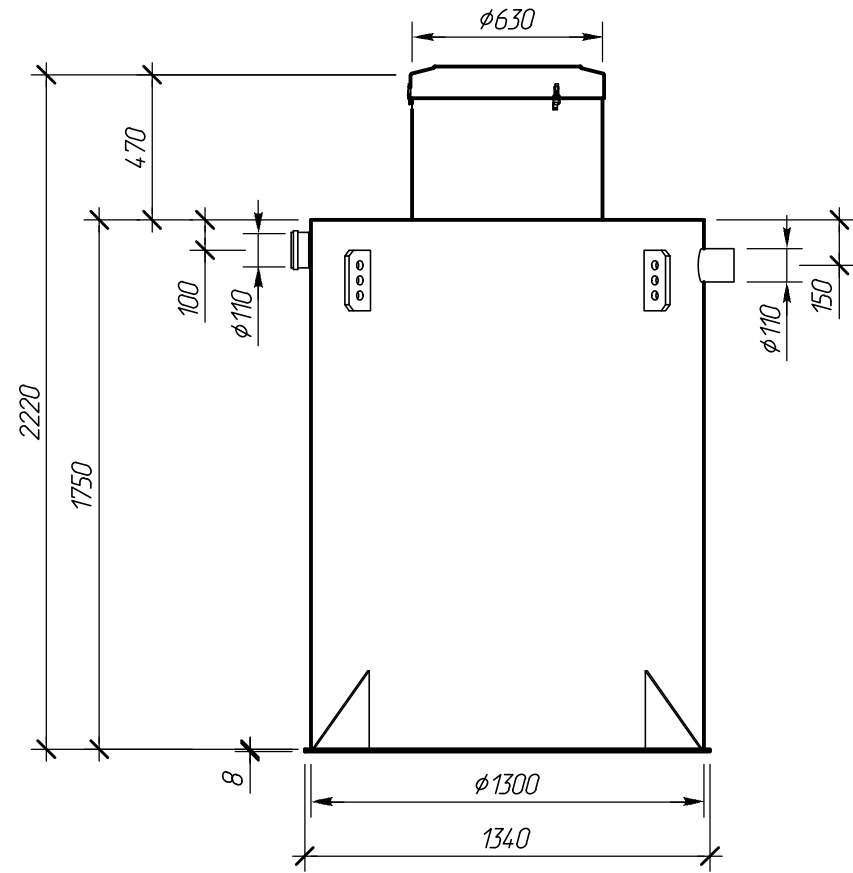
Вид спереди
