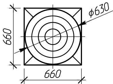
Вид сверху
