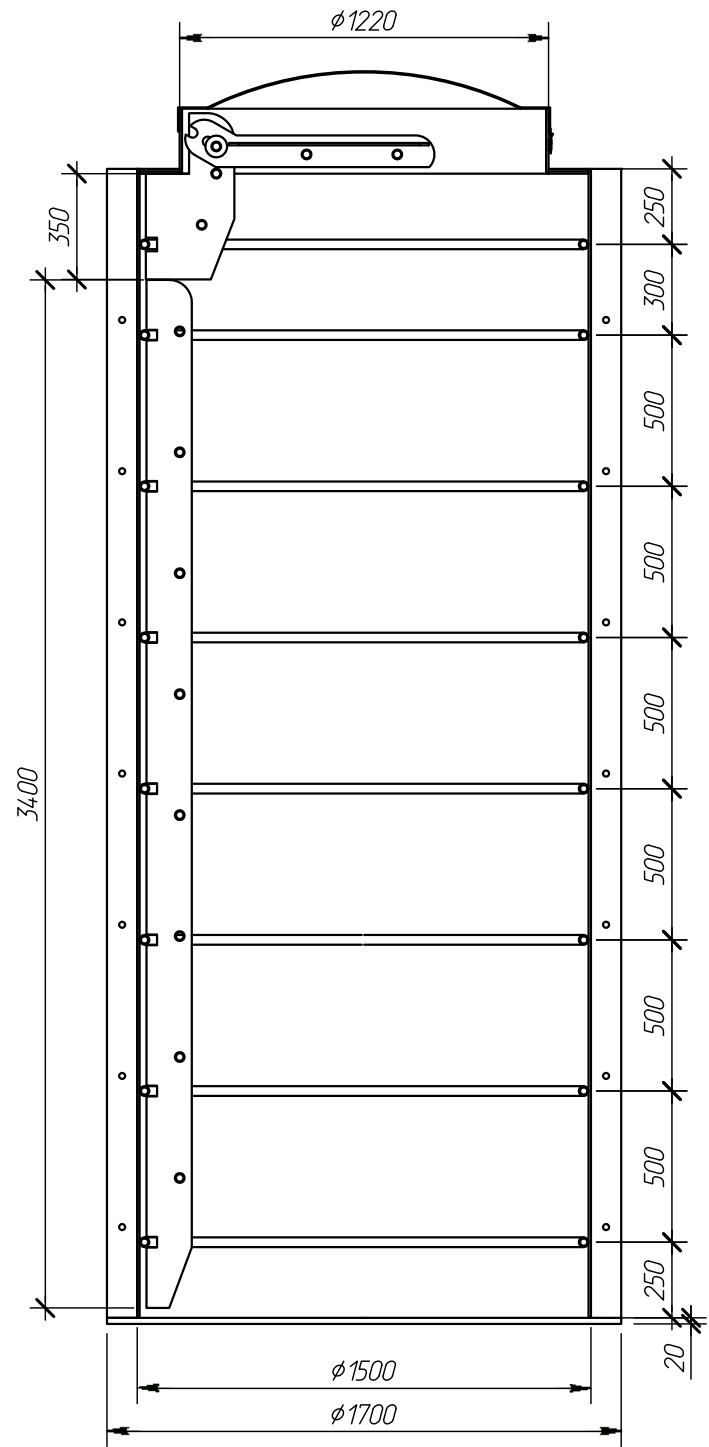
Разрез А-А
