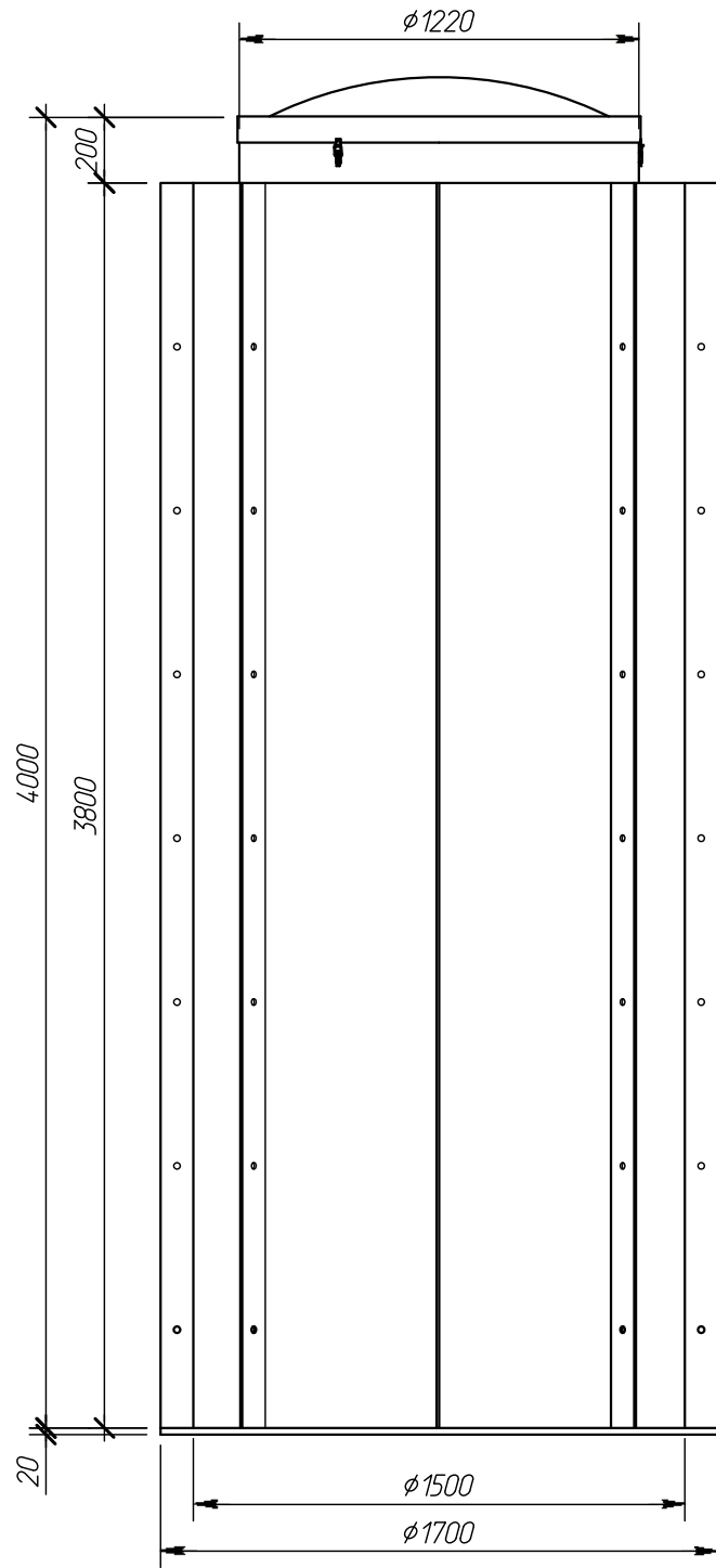
Вид спереди
