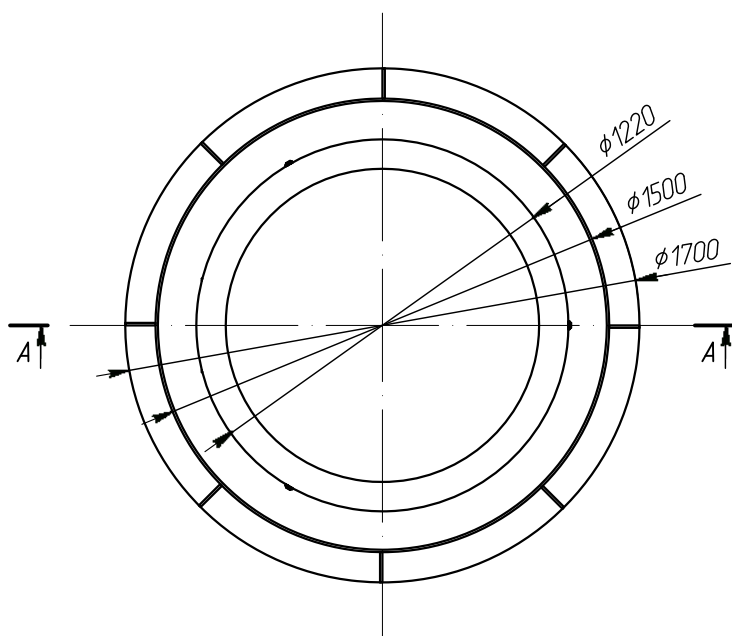
Вид сверху
